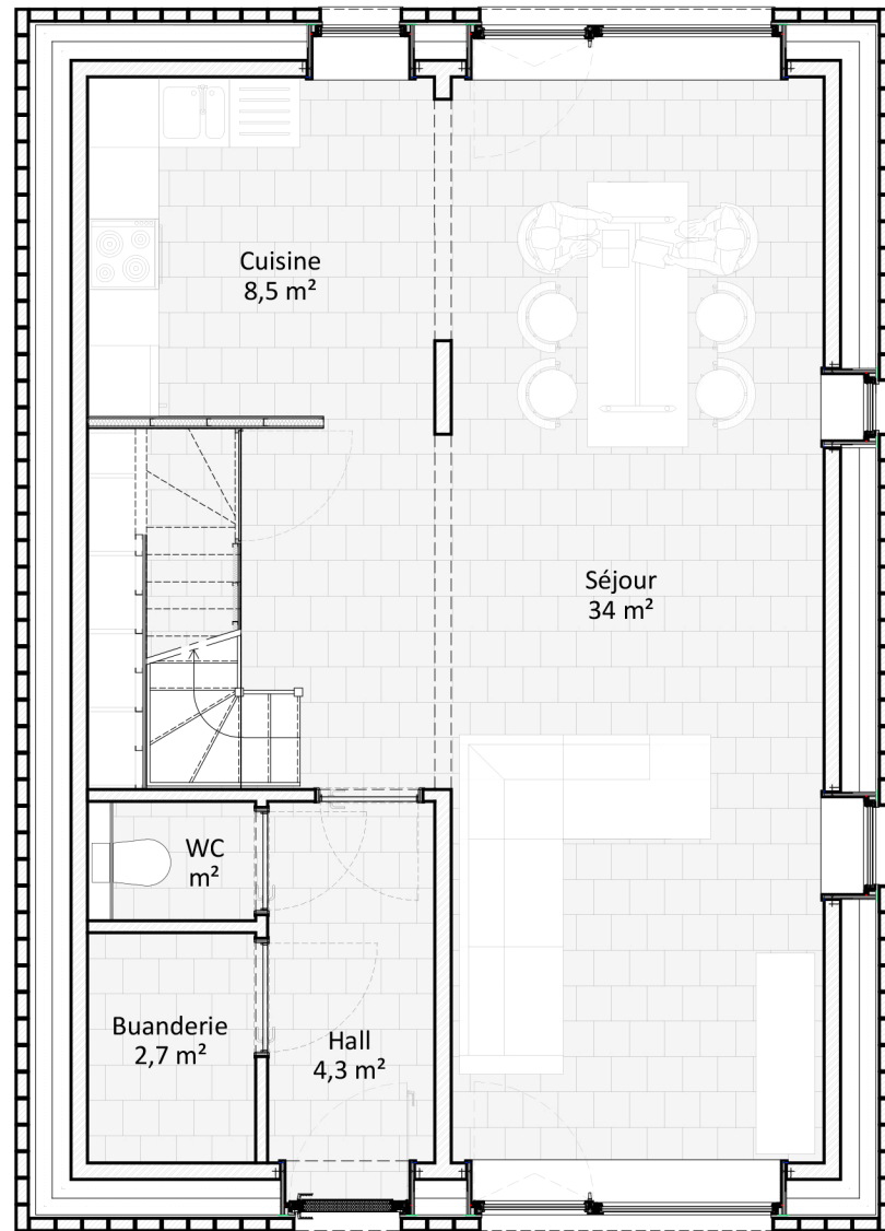
REZ-DE-CHAUSSÉE
