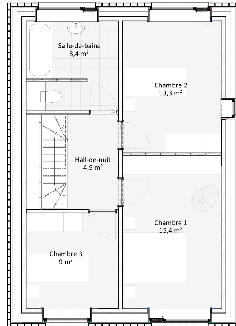
ÉTAGE
